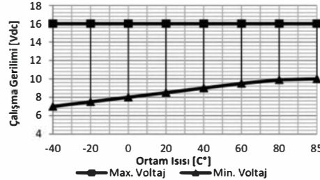
Min. ve Max. Çalışma Gerilimi
