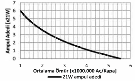
Ortalama Ürün Ömrü
