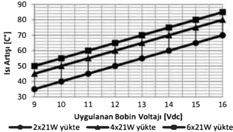
Çalışma Voltajına Göre Isı Artışı
